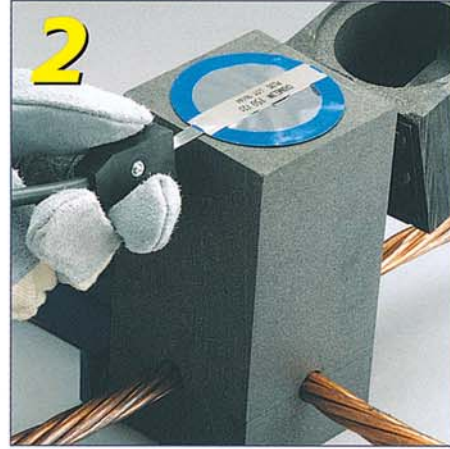
Adım 2: Ateşleme şeridine elektronik ateşleyici bağlanır.
